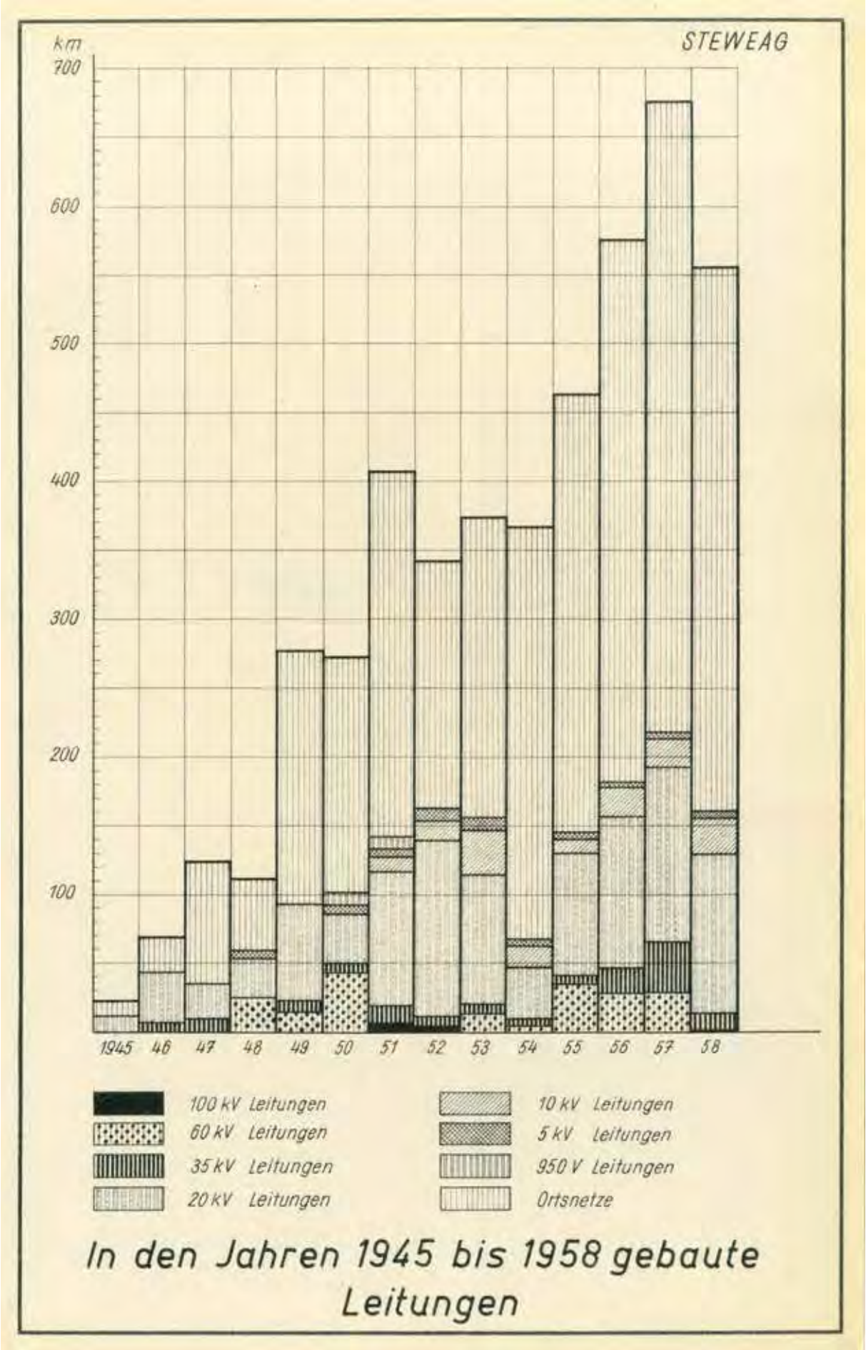
Die Nachkriegsleistung der STEWEAG: Der Leitungsbau 1945–1958
