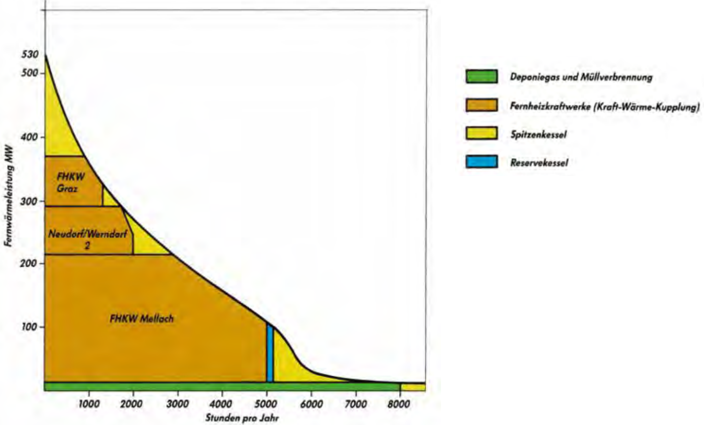
Die Deckung des Bedarfs an Fernwärme durch die STEWEAG 1988
