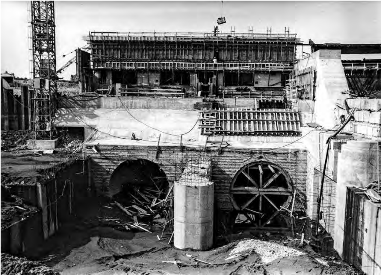
Auslauf der zwei Rohrturbinen im Krafthaus Gabersdorf
