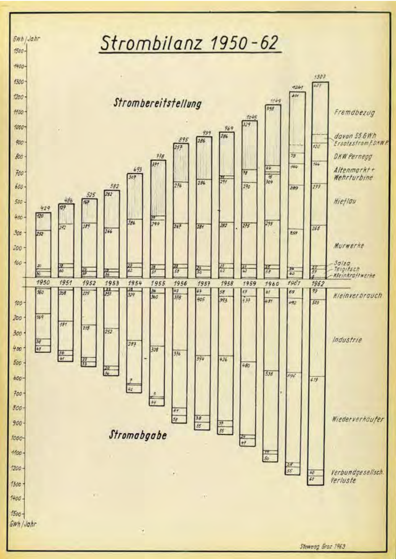
Strombereitstellung und Stromabgabe der STEWEAG 1950–1962
