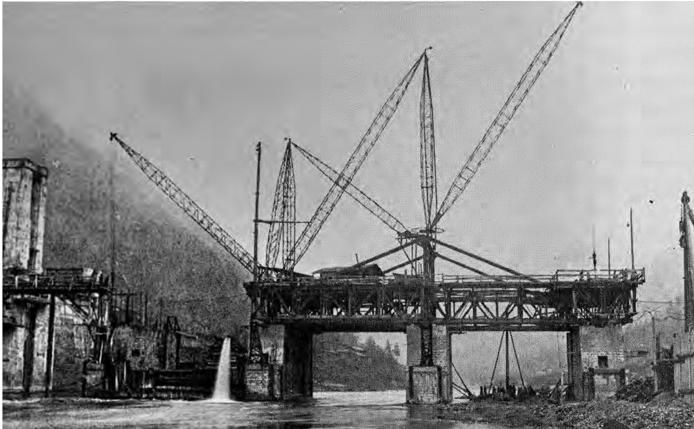
Das Kraftwerk Faal/Fala während der Bauarbeiten 1916
