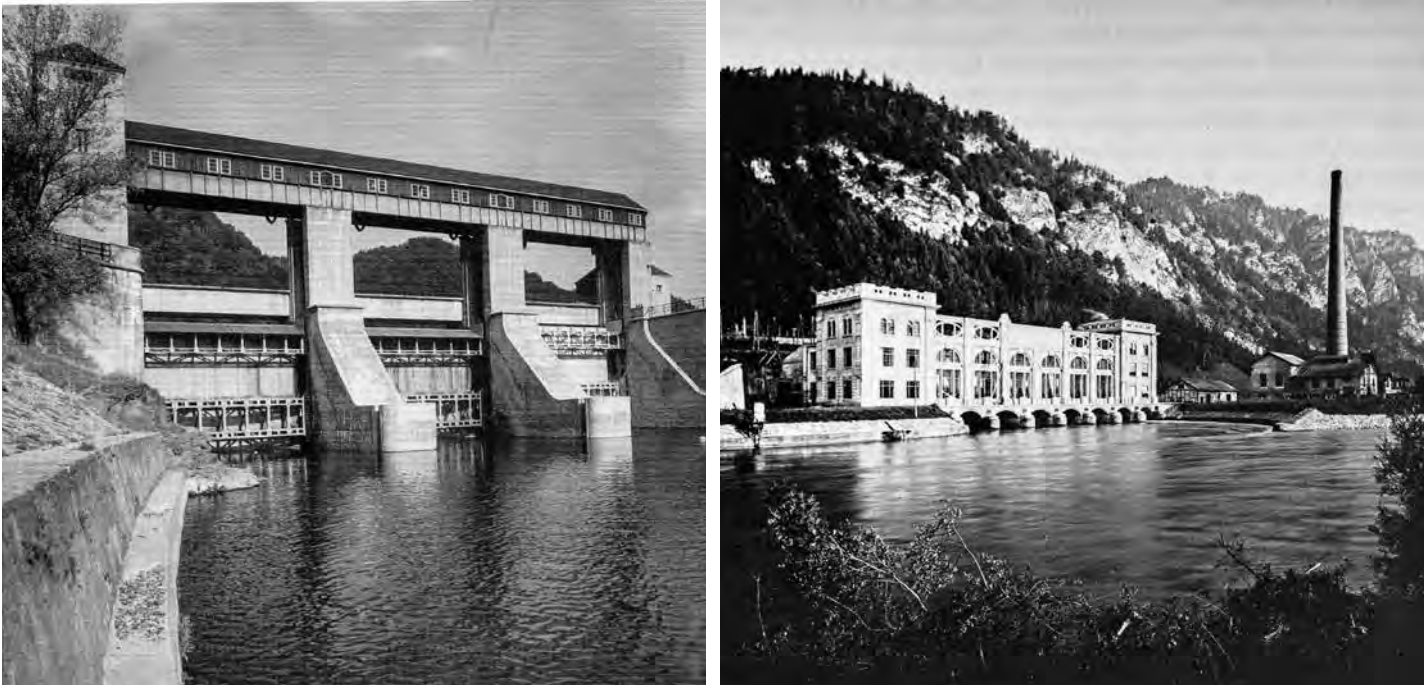
Außenansichten der Kraftwerke Pernegg und Peggau (rechts). Zeugnisse aufwendiger Industriearchitektur zu Beginn des 20. Jahrhunderts
