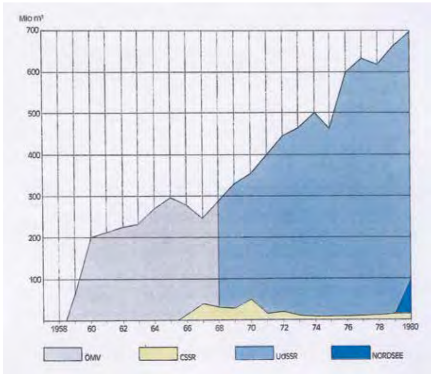
Die Erdgasabgabe der Steirischen Ferngas und die Herkunft des Erdgases 1960 bis 1980
