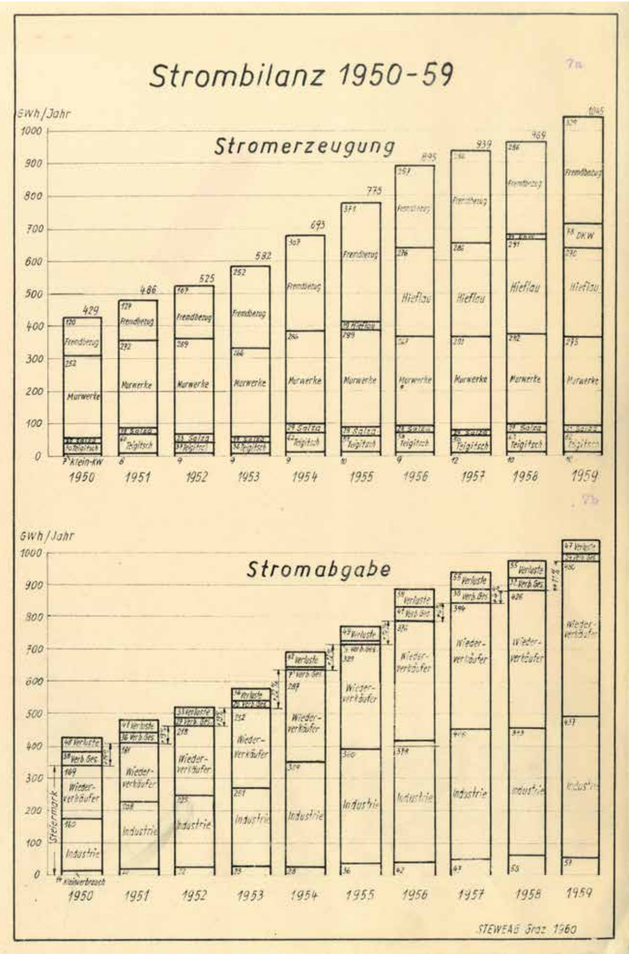
Die Stromerzeugung der STEWEAG-Kraftwerke 1950–1959
